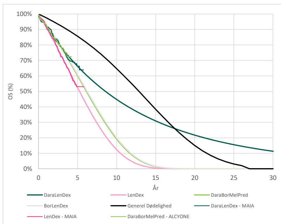
Figur 6. Ansøgers ekstrapolerede OS-kurver for alle behandlingsregimer baseret på HR fra NMA og data fra MAIA-studiet. Det er ikke muligt at se DaraBorMelPred og DaraLenDex, da kurven fra BorLenDex dækker.
