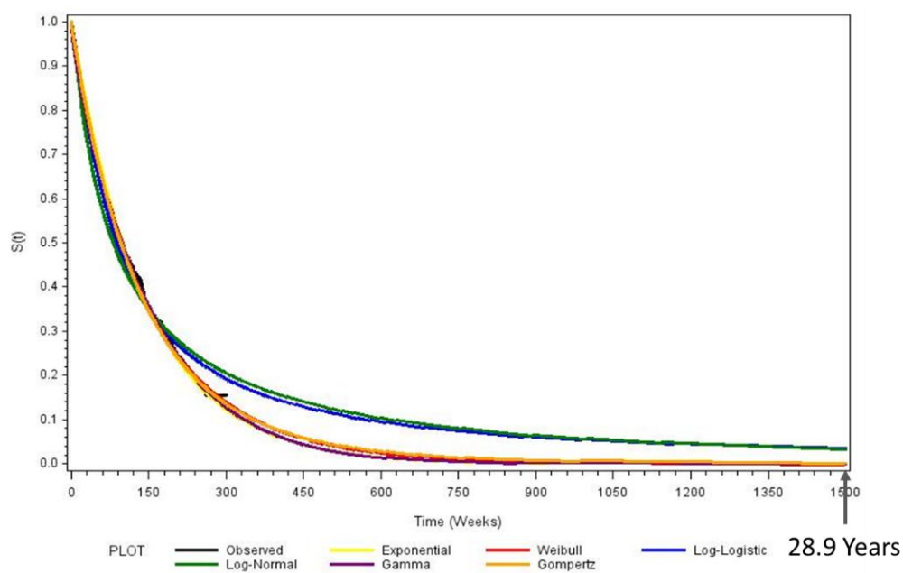
Bilag B-7. Ekstrapolering af behandlingsvarigheden for LenDex
