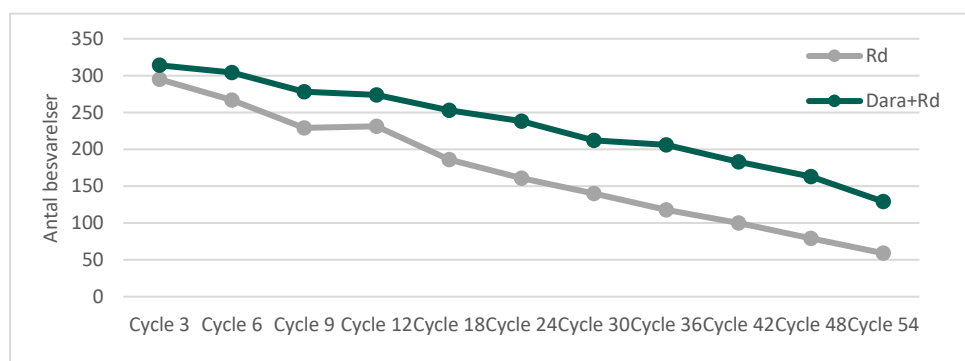
Figur 13. Antal af EORTC QLQ-C30 besvarelser (MAIA)
