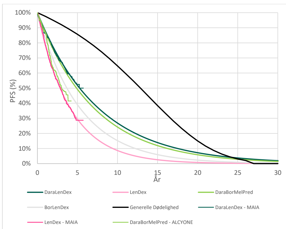
Figur 11. Ansøgers ekstrapolerede PFS-kurver for alle behandlingsregimer, 1. linje, baseret på studiedata og HR fra NMA og PFS-data fra MAIA
